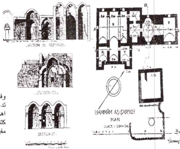
(شكل-٨) المسقط الاقي و قطاعات لحمام الصرخ . بشرق الأردن عام ٧٢٥-٧٣٠ م المصدر : كمال الدين سامح - العمارة في صدر الإسلام ١٩٨٧ م
