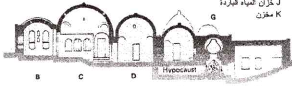
(شكل-٢٤) مسطق أفقي و قطاع لحمام شكر بصنعاء باليمن ١٥٩٨ م . المصدر :
