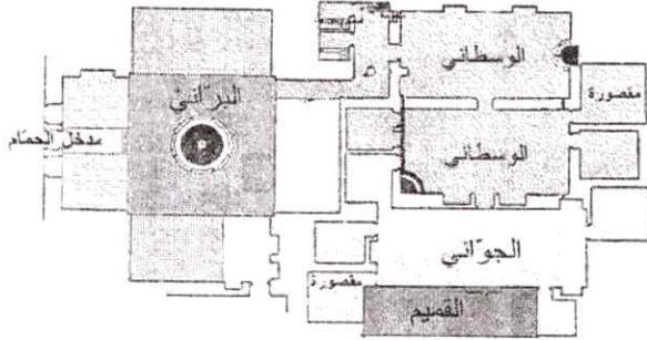
(شكل-٢٩) رسم كروكي لإيضاح المناطق المختلفة للحمام الدمشقي القديم - حمام بليغا الناصري و هو من أهم حمامات سورية . المصدر : http://www.discover-syria.com/results/114
