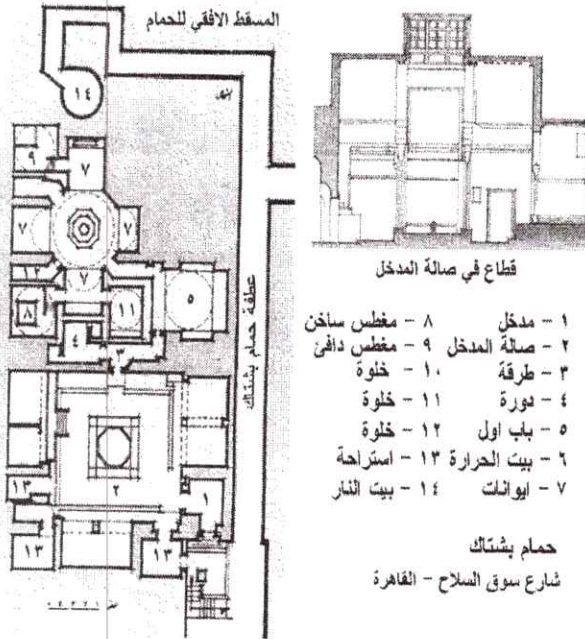
(شكل-٢٠) مسقط أفقي لحمام بشتاك وقطاع في صالة المدخل .
