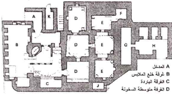
مسقط أفقي وقطاع لحمام شكر بصنعاء (١٥٩٨م-١٠٠٧هـ)
