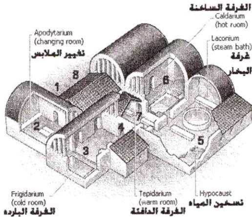
(شكل-٢) شرح مبسط لمكونات و مراحل الحمام الروماني . حيث يعبر التسلسل الرقمي عن مراحل الحمام المختلفة . المصدر :
