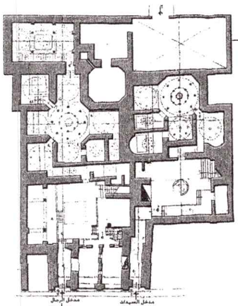
(شكل-٣٢) المسقط الافقي لحمام الملاطيلي - و يظهر تخصيص جزء من الحمام لاستخدام السيدات و جزء اخر للرجال و وجود مدخلين للحمام . المصدر : عاصم محمد رزق - اطلس العمارة الاسلامية و القبطية بالقاهرة - مكتبة مندوبلي - ٢٠٠٤ .
