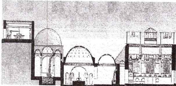
طريقة تغذية المغطس و الحنفيات بالمياه في الحمامات الشعبية
