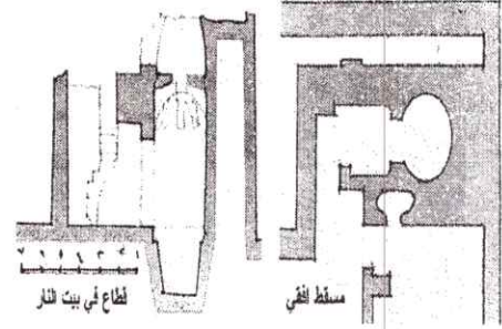
(شكل-٢٢) مسطق أفقي و قطاع في بيت النار ( الجورة ) بالحمامات الشعبية القديمة. المصدر: عاطف فهيم - الحمامات الشعبية في مصر - ١٩٧٥م.
