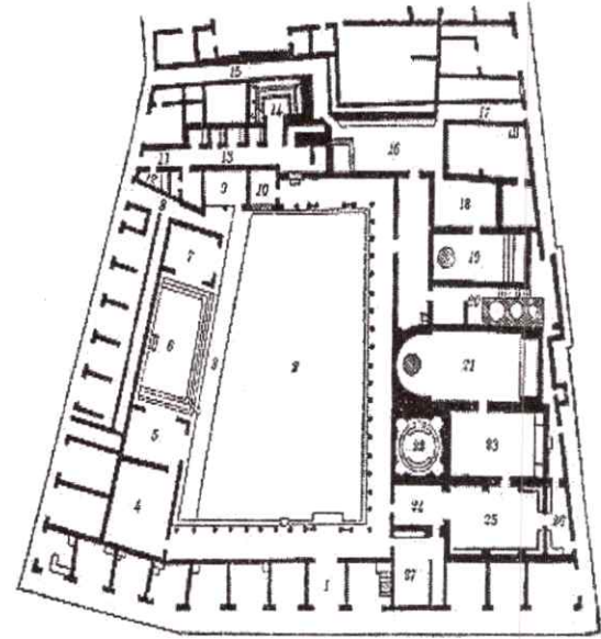
(شكل-٢٨) المسقط الأثني لحمام ستبان بومباي . PLAN OF THE STABIAN BATHS AT POMPEII المصدر :
