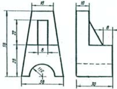
المسقط الرأسي
