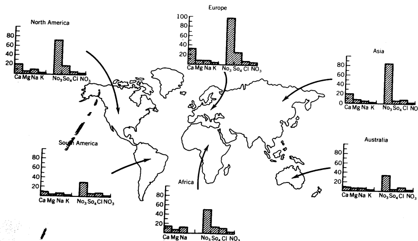
الشكل (4) : متوسط تركيز الكاتيونات والأنيونات في المياه العذبة في العالم
