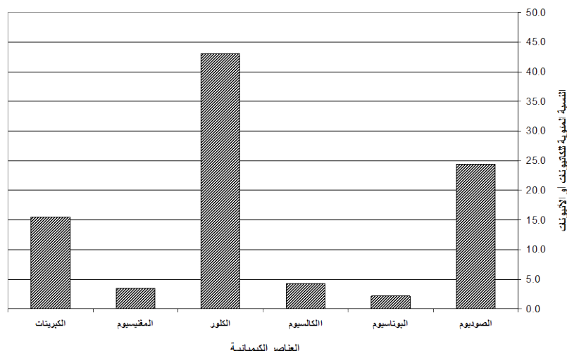
الشكل (5): النسبة المئوية لتركيز الأيونات لمياه عين الخدود .
